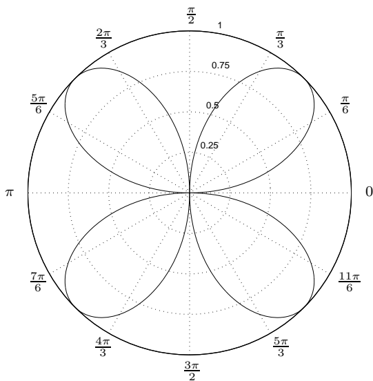
r = \sin 2\theta (Rose)
