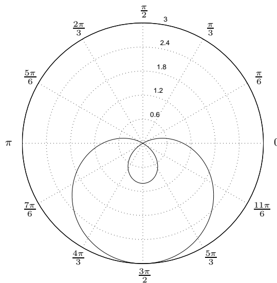
r = 1 - 2 \sin \theta (Limaçon)
